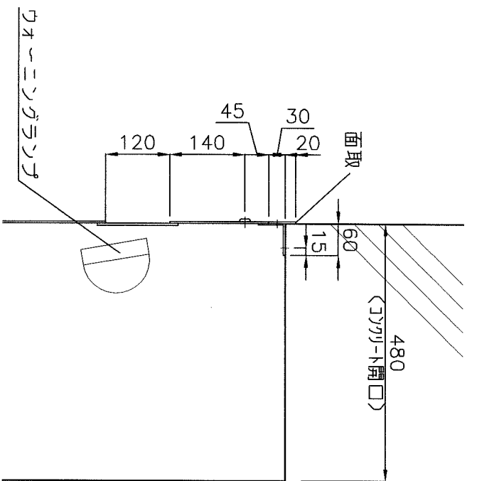
コロボ断面図 1:10
