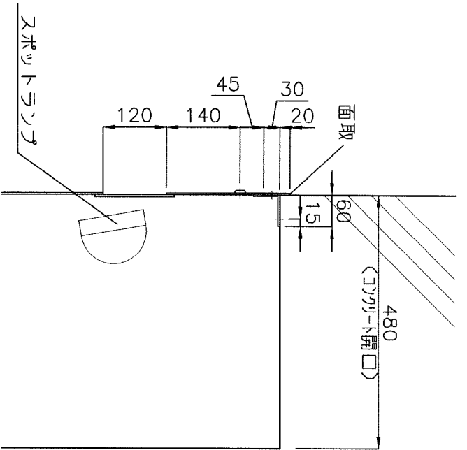
ク拡大図 1:10
